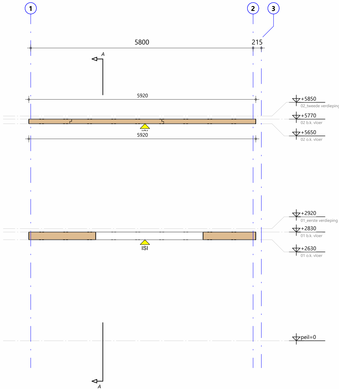
Doorsnede B , Schaal: 1 : 50
